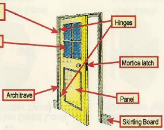
Internal Door
