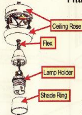
Lighting Pendant
